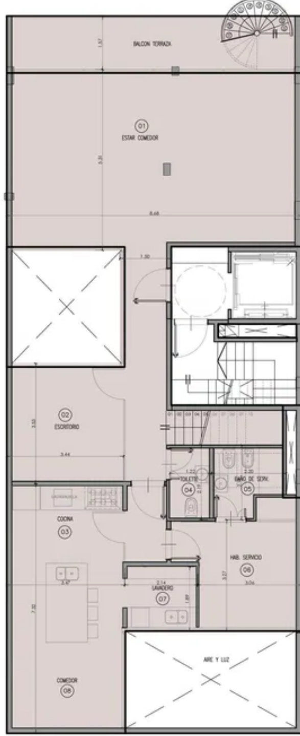
PLANTA 9° PISO
